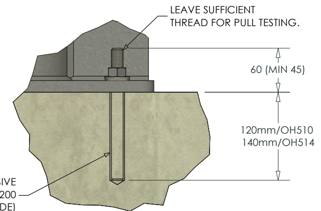
DETAIL A ( 1 : 5 )
