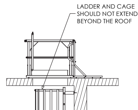
SECTION A-A ( 1 : 60 )
