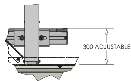
DETAIL Z ( 1 : 10 )
