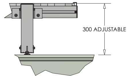
DETAIL Z ( 1 : 10 )
